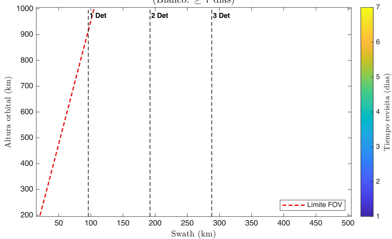
Tiempo Revisita - 1 Satellite(s); 2 Telescopio(s): Cassegrain; Detector 1 (Blanco: \geq 7 dias)
